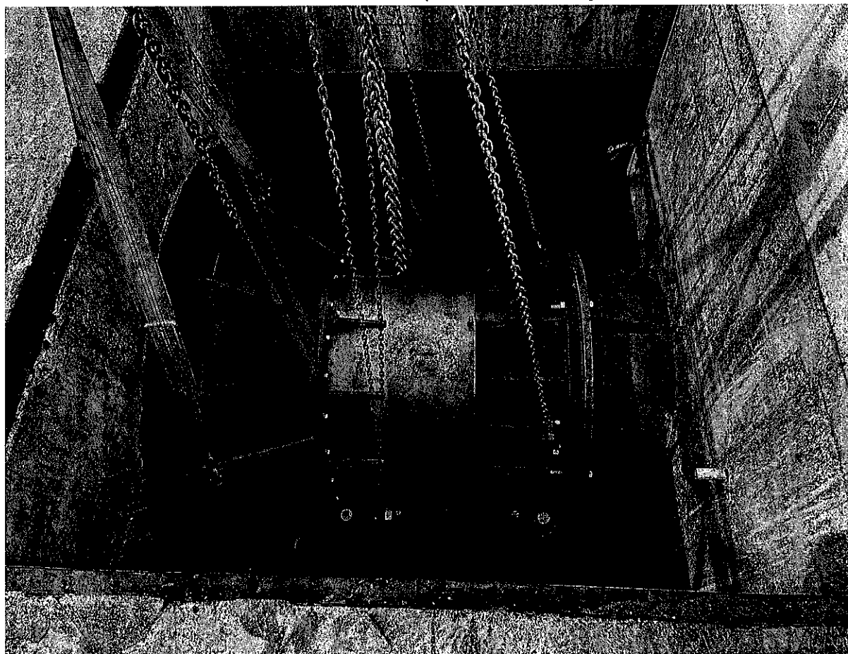
слика 2 - приказ на конусен вентил Howell Bunger
